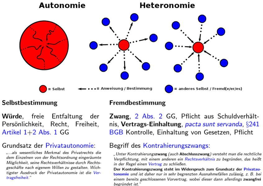
Abbildung 1: Das nomische Gleichgewicht
